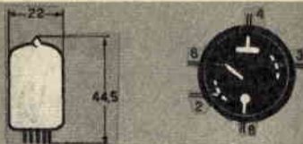
Fig. 2 - L'intero complesso necessario per ottenere il controllo di fiamma può essere racchiuso in una piccola scatola metallica in cui verrà praticata un'apertura che permetterà di colpire la fotoresistenza nella sua parte sensibile. Nella figura, in alto, sono riportate le dimensioni della valvola Trigger e la numerazione dei terminali sullo zoccolo.
