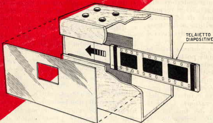
Fig.1 - La scatola del proiettore può essere costruita in legno o cartone. Le diapositive sono contenute in un telaietto costituito da due lastre di vetro, il cui spessore dev'essere uguale a quello della larghezza delle guide di scorrimento.
