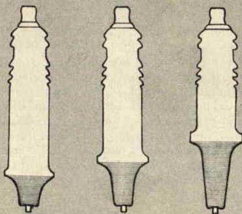
Fig. 1 - La temperatura della candela non è mai uniforme in ogni suo punto, la più critica è quella riguardante gli elettrodi che devono mantenersi, per ogni candela, in qualsiasi condizione di lavoro, tra i 500 e i 900 gradi centigradi.
