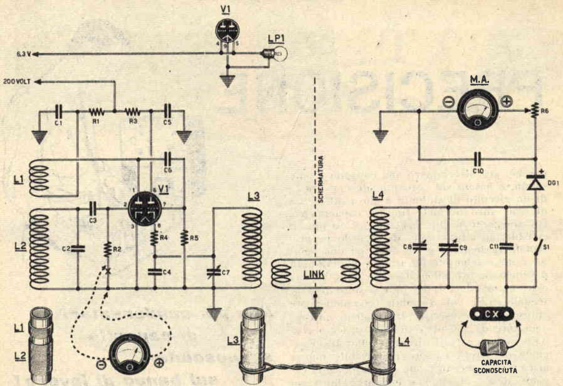
Fig. 2 - Il circuito elettrico del capacimetro è alquanto semplice: esso è costituito da un circuito oscillatore a frequenza fissa e da un circuito di sintonia in cui viene inserito il condensatore (CX) di cui si vuol conoscere l'esatto valore capacitivo.
